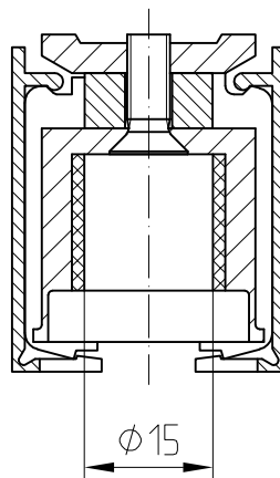
Schnitt A-B
