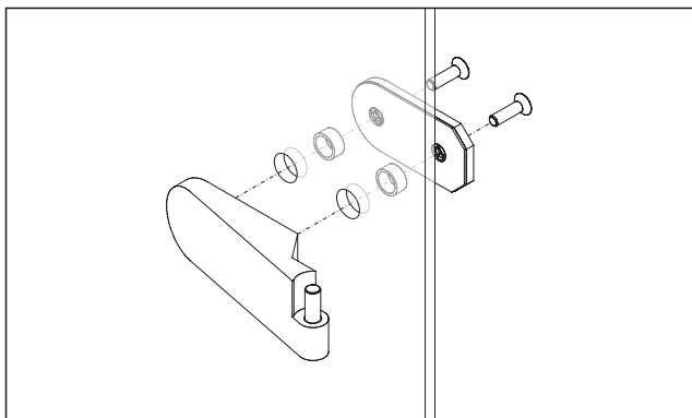
Abb. 3 Rahmenteil montieren
